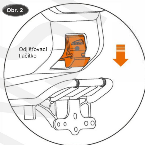
Zadní strana
